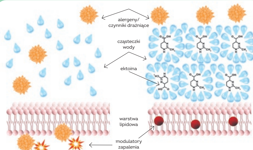
Rycina 1. Schemat działania ektoiny na nabłonek błon śluzowych.
